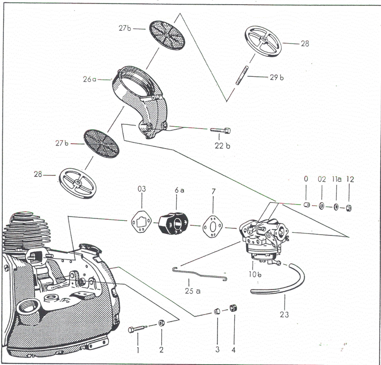
Bildtafel F Vergaser, Filterstutzen, Luftfilter
